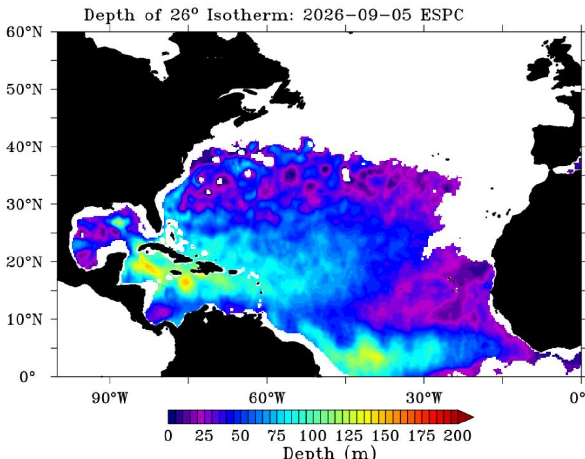
FIGURA 60. Variación en la extensión espacial de la profundidad de la isoterma oceánica de 26°C. Fuente: https://www.ospo.noaa.gov/Products/ocean/ohc/ (accedido: 5 de septiembre de 2026).
