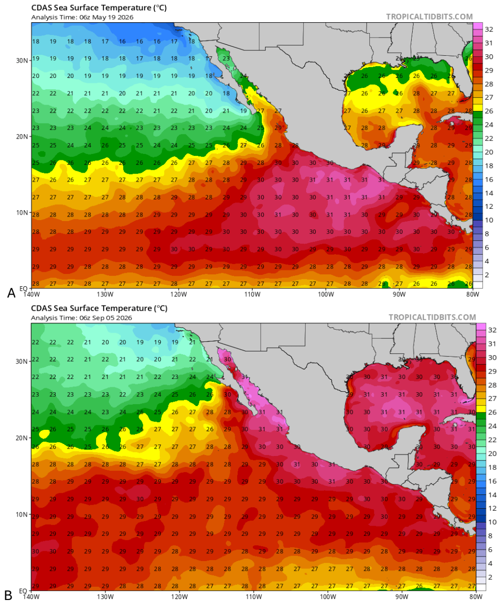
FIGURA 10. Patrones de distribución de temperaturas superficiales del mar en el este del Pacífico tropical. Accedido: A) 19 de mayo de 2026; B) 5 de septiembre de 2026. Fuente: https://www.tropicaltidbits.com/analysis/ocean/cdas-sflux_sst_epac_1.png
