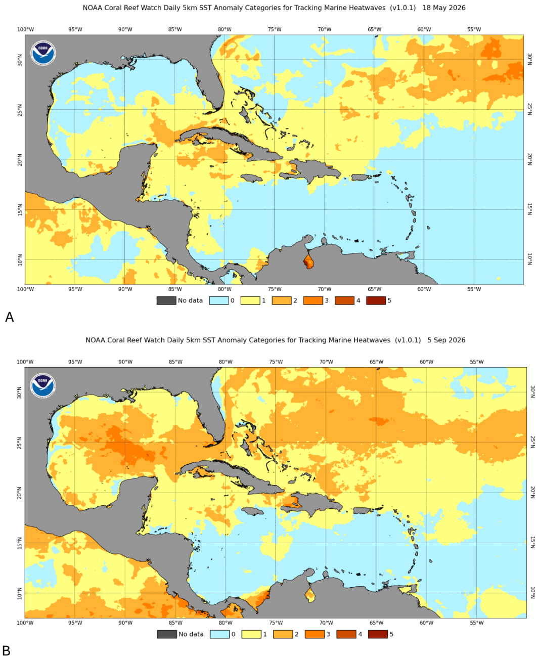
FIGURA 15. Clasificación actual del NOAA Coral Reef Watch Program de la ola de calor marino atravesando la zona del Caribe. Accedido: A) 19 de mayo de 2026; B) 5 de septiembre de 2026. Fuente: https://coralreefwatch.noaa.gov/data_current/marine_heatwave/v1.0.1/daily/png/noaa-crw_mhw_v1.0.1_category_caribbean_current.png
