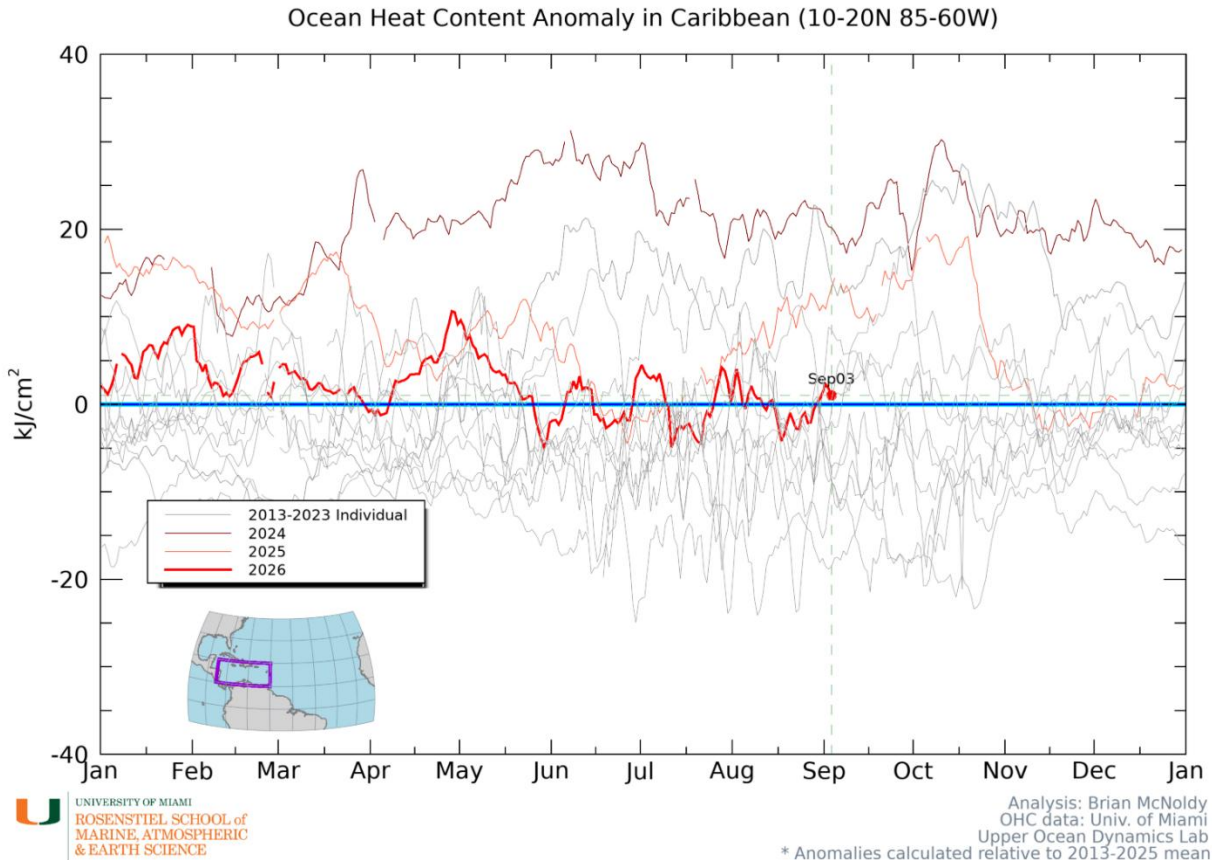
FIGURA 56. Anomalía del contenido de calor oceánico para el Caribe. (accedido: 5 de septiembre de 2026). Fuente: https://bmcnoldy.earth.miami.edu/tropics/ohc/ohc_carib_anom.png
