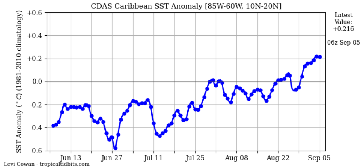
FIGURA 20. Patrones de variación reciente en la anomalía térmica del mar en la región del Mar Caribe. Fuente: https://www.tropicaltidbits.com/analysis/ocean/carssta.png (accedido: 5 de septiembre de 2026).
