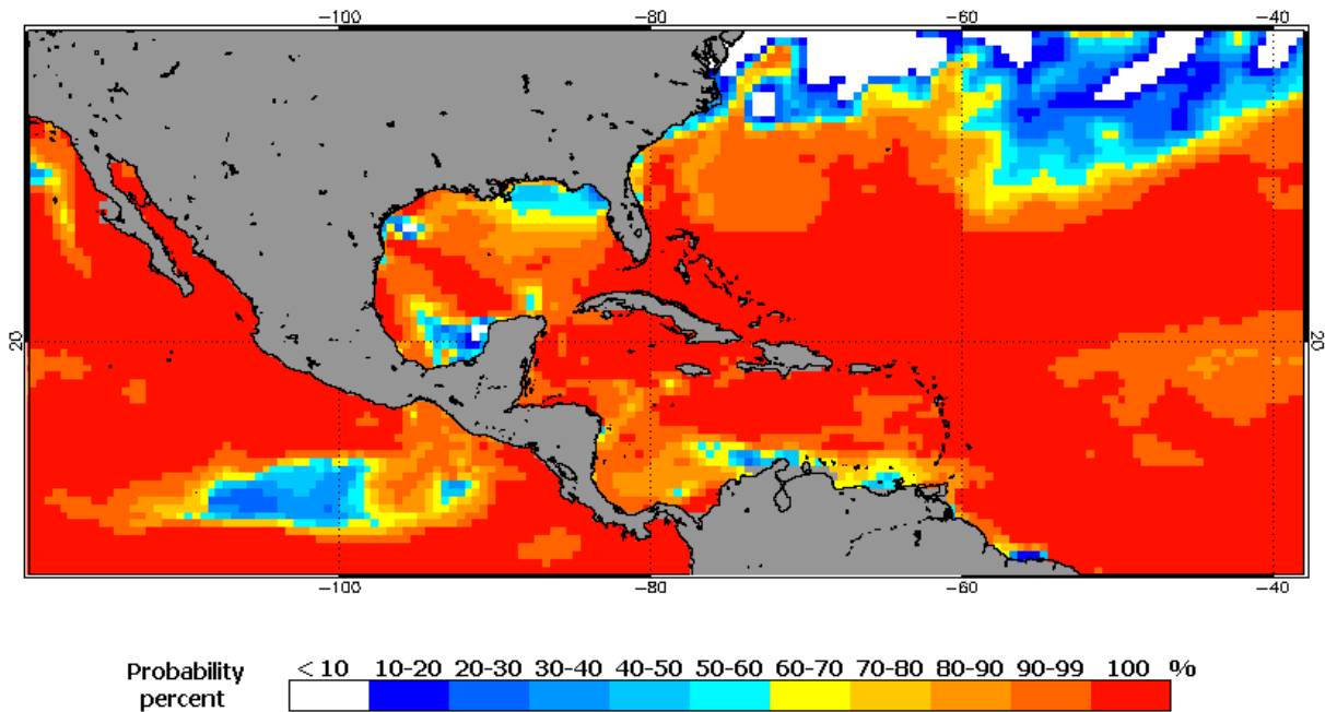
FIGURA 51. Proyección de probabilidad de emisión de al menos un aviso o mayor de blanqueamiento inminente de los corales en el Caribe para el período septiembre a diciembre de 2026. Accedido: 5 de septiembre de 2026. Fuente: https://coralreefwatch.noaa.gov/satellite/bleachingoutlook_cfs/current_image/cur_cfsv2_prob-4mon_v5_warning_caribbean.gif
