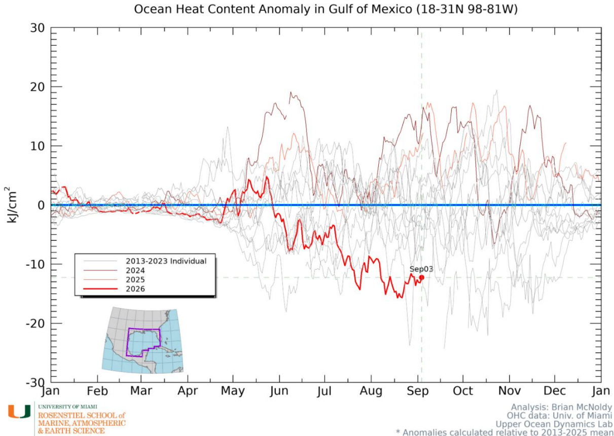
FIGURA 58. Anomalía del contenido de calor oceánico para el Golfo de México. (accedido: 5 de septiembre de 2026). Fuente: https://bmcnoldy.earth.miami.edu/tropics/ohc/ohc_gulf_anom.png
