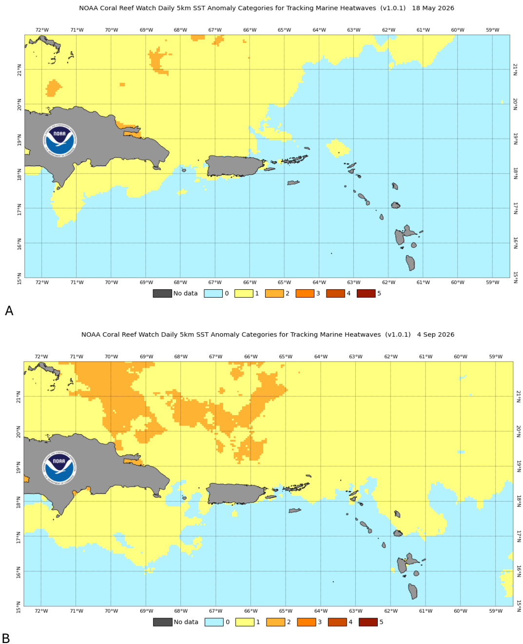
FIGURA 16. Clasificación actual del NOAA Coral Reef Watch Program de la ola de calor marino atravesando la zona de Puerto Rico. Accedido: A) 19 de mayo de 2026; B) 5 de septiembre de 2026. Fuente: https://coralreefwatch.noaa.gov/data_current/marine_heatwave/v1.0.1/daily/png/noaa-crw_mhw_v1.0.1_category_prusvi_current.png
