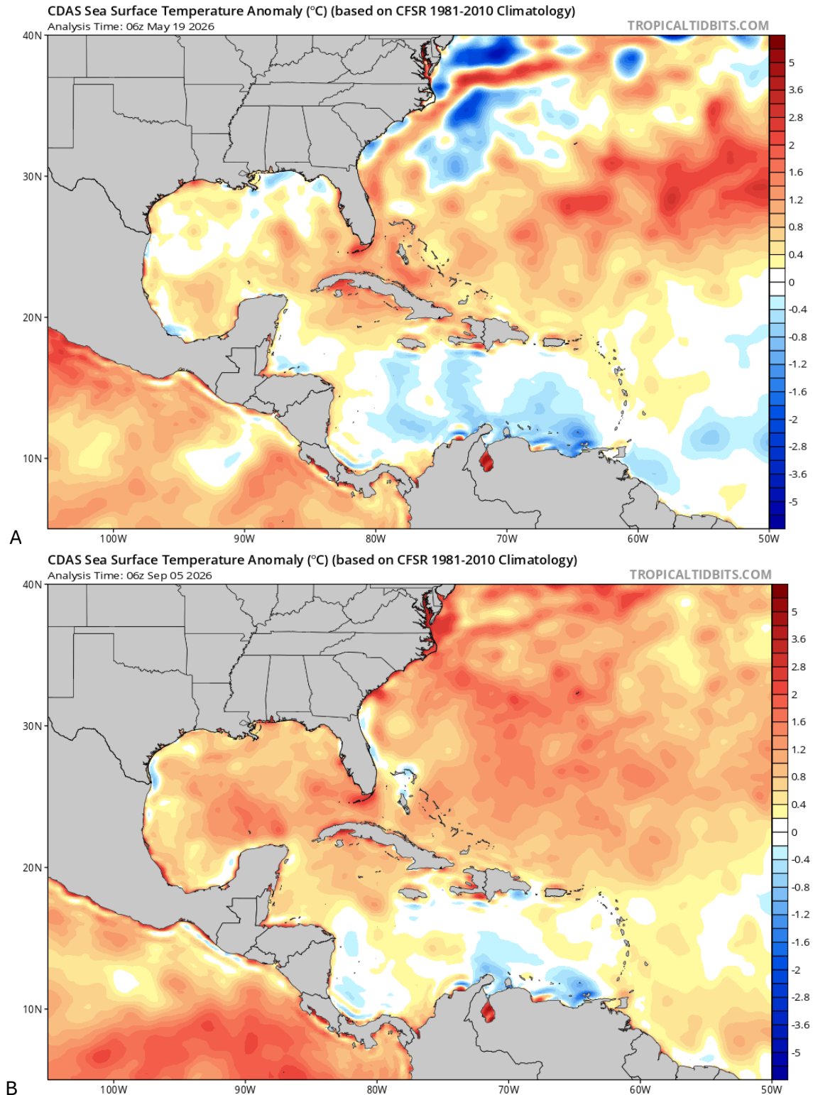
FIGURA 13. Patrones de distribución de las anomalías térmicas en la superficie del mar a través del Mar Caribe. Accedido: A) 19 de mayo de 2026; B) 5 de septiembre de 2026. Fuente: https://www.tropicaltidbits.com/analysis/ocean/cdas-sflux_ssta_watl_1.png
