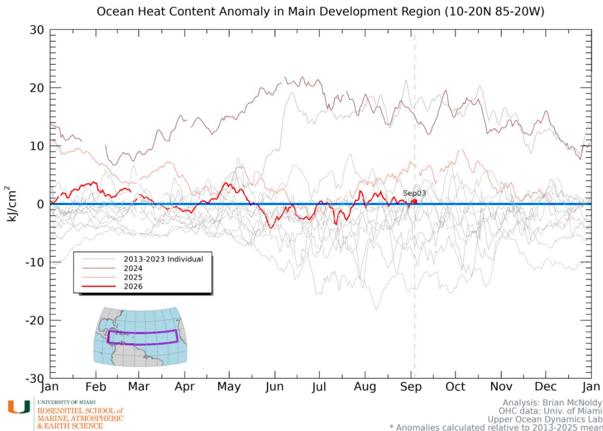
FIGURA 55. Anomalía del contenido de calor oceánico para el Atlántico tropical y el Caribe. (accedido: 5 de septiembre de 2026). Fuente: https://bmcnoldy.earth.miami.edu/tropics/ohc/ohc_mdr_anom.png
