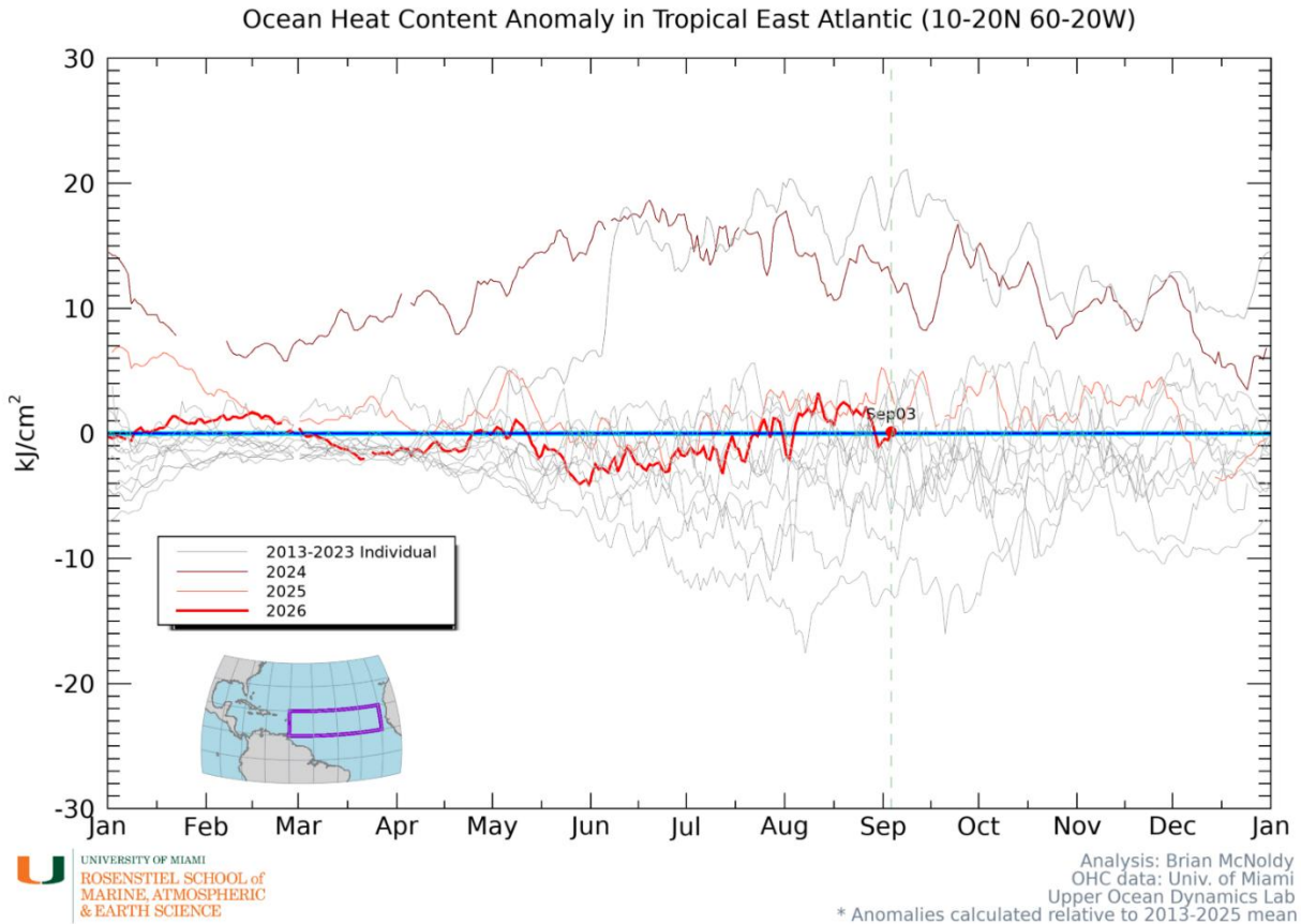
FIGURA 57. Anomalía del contenido de calor oceánico para el este del Atlántico tropical. (accedido: 5 de septiembre de 2026). Fuente: https://bmcnoldy.earth.miami.edu/tropics/ohc/ohc_east_anom.png
