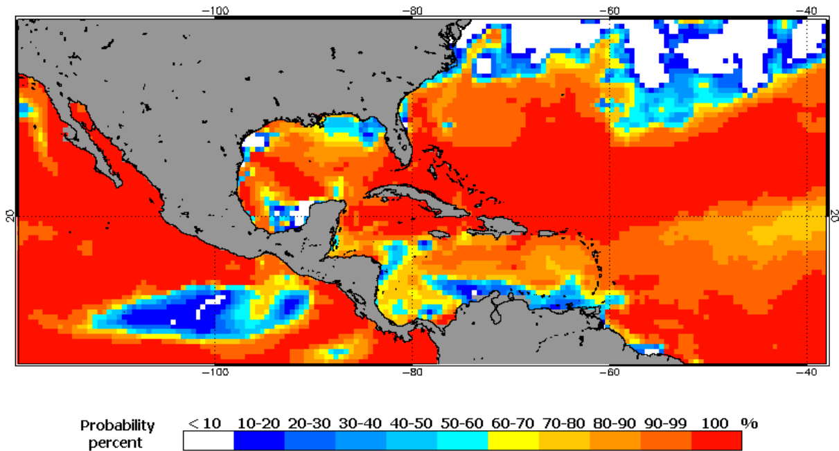
FIGURA 50. Proyección de probabilidad de emisión de una alerta de nivel 1 o 2 de blanqueamiento inminente de los corales en el Caribe para el período de septiembre a diciembre de 2026. Accedido: 5 de septiembre de 2026. Fuente: https://coralreefwatch.noaa.gov/satellite/bleachingoutlook_cfs/current_image/cur_cfsv2_prob-4mon_v5_alertlevel1_caribbean.gif
