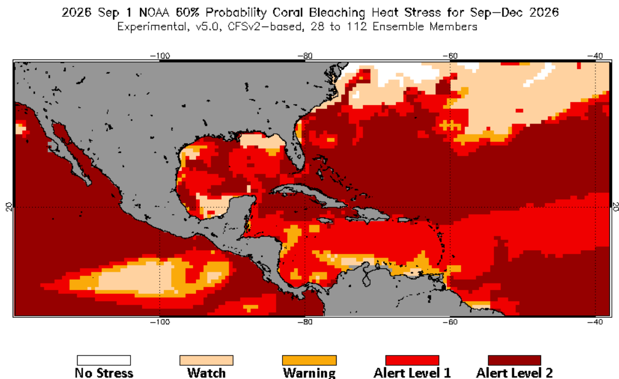
FIGURA 48. Proyección de probabilidad de 60% o mayor de estrés térmico conducente al blanqueamiento de los corales en el Caribe para el período de septiembre a diciembre de 2026. Accedido: 5 de septiembre de 2026. Fuente: https://coralreefwatch.noaa.gov/satellite/bleachingoutlook_cfs/current_image/cur_cfsv2_outlook-4mon_v5_60pct_caribbean.gif
