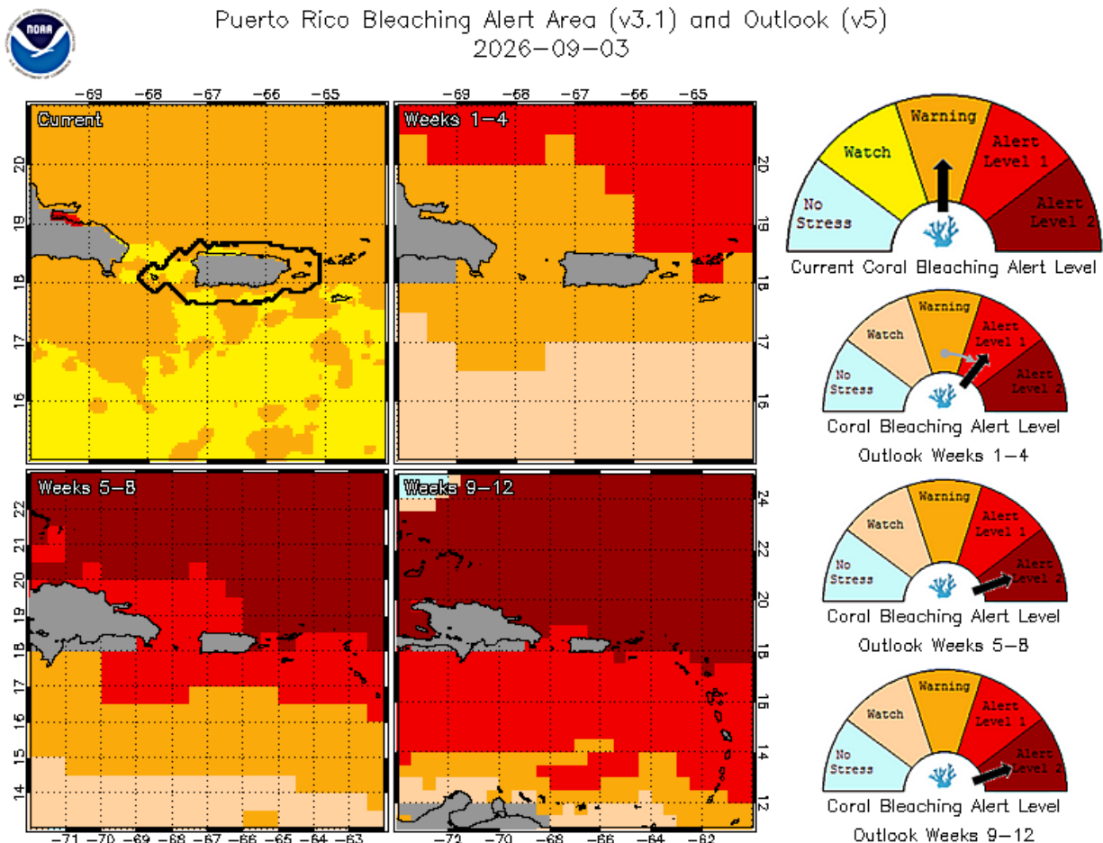
FIGURA 43. Proyecciones potenciales de las alertas de blanqueamiento para Puerto Rico para los meses de septiembre a noviembre de 2026. Fuente: https://coralreefwatch.noaa.gov/product/vs/gauges/puerto_rico.php (accedido: 5 de septiembre de 2026).
