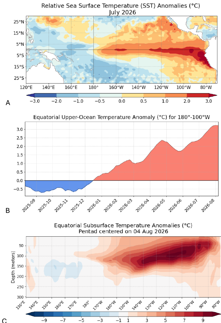
FIGURA 7. A) Anomalías térmicas (°C) en la superficie del mar en el Pacífico Tropical; B) Anomalías térmicas (°C) subsuperficiales (0-300 m) de las regiones de El Niño en el Océano Pacífico; C) Variación longitudinal en las anomalías térmicas (°C) subsuperficiales (0-300 m) de las regiones de El Niño en el Océano Pacífico. Las anomalías se calcularon contra la base histórica de datos de 1991-2020 utilizando los promedios semanales. Fuente: https://www.cpc.ncep.noaa.gov/products/analysis_monitoring/enso_advisory/ (Accedido: 5 de agosto de 2026).
