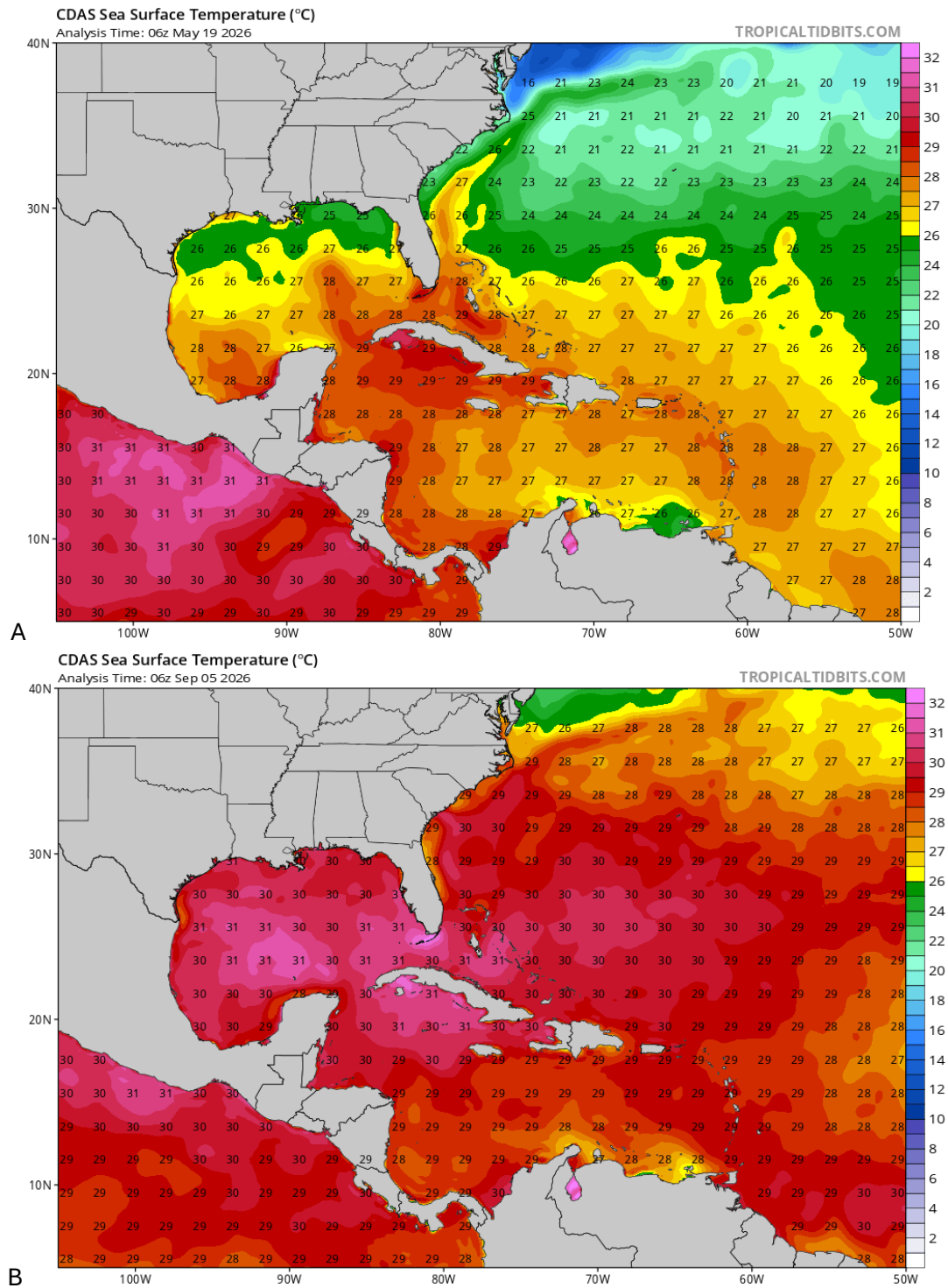
FIGURA 12. Patrones de distribución de temperaturas superficiales del mar a través del Mar Caribe. Accedido: A) 19 de mayo de 2026; B) 5 de septiembre de 2026. Fuente: https://www.tropicaltidbits.com/analysis/ocean/cdas-sflux_sst_watl_1.png
