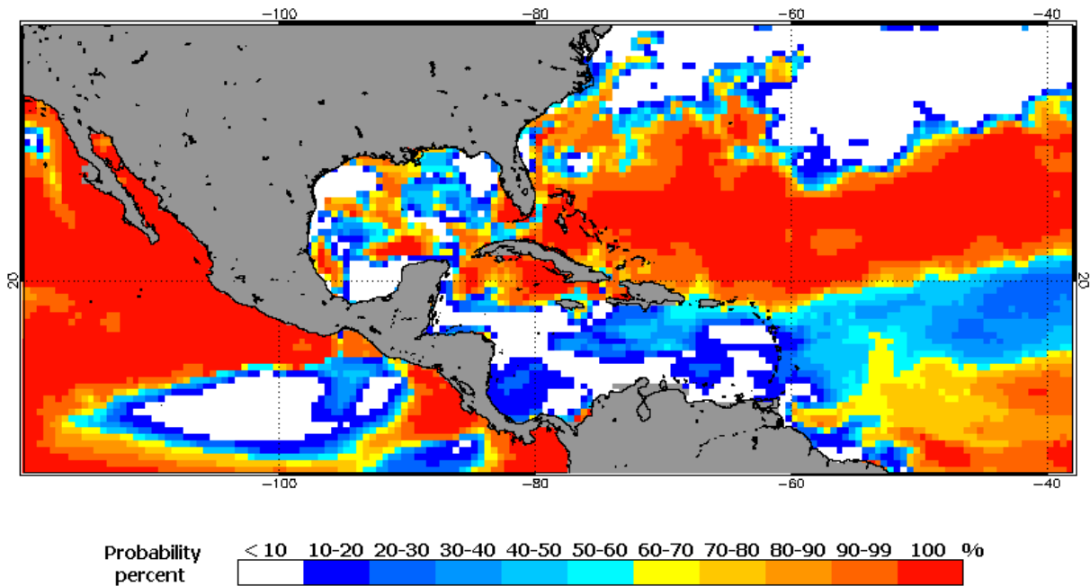
FIGURA 49. Proyección de probabilidad de emisión de una alerta de nivel 2 de blanqueamiento inminente de los corales en el Caribe para el período de septiembre a diciembre de 2026. Accedido: 5 de septiembre de 2026. Fuente: https://coralreefwatch.noaa.gov/satellite/bleachingoutlook_cfs/current_image/cur_cfsv2_prob-4mon_v5_alertlevel2_caribbean.gif
