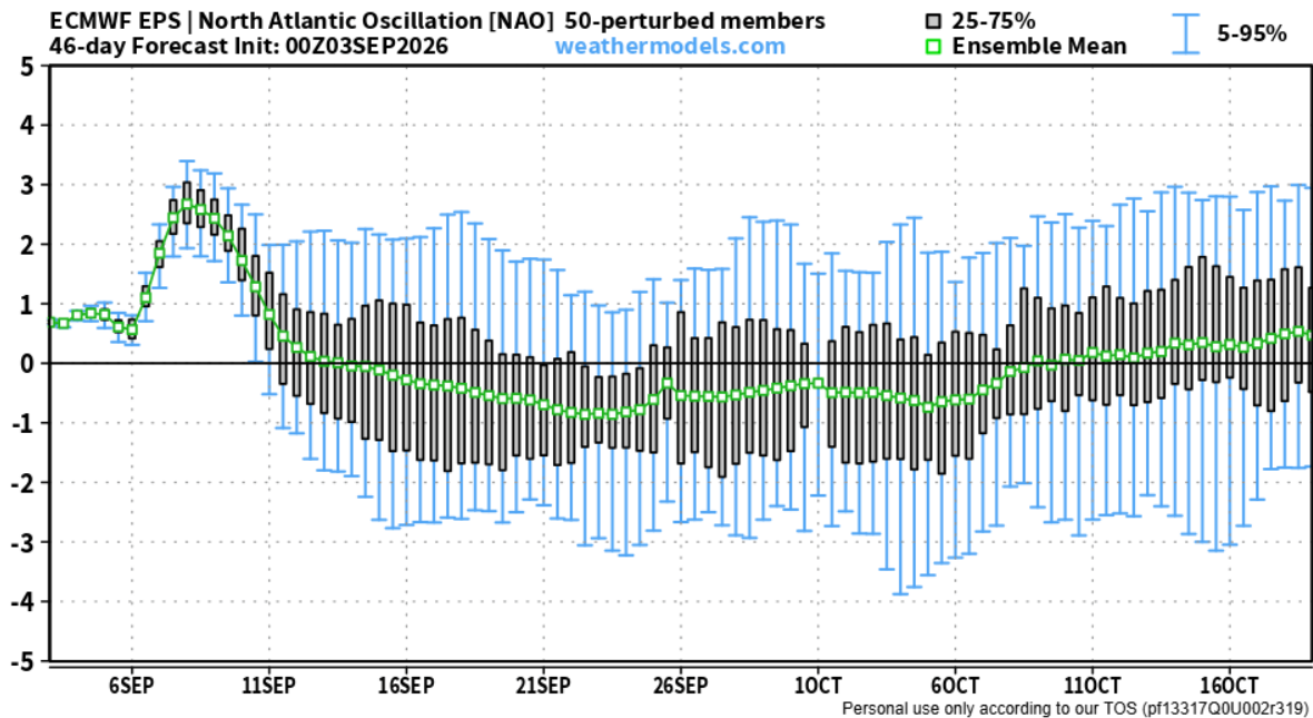
FIGURA 61. Oscilación del Atlántico Norte (NAO) para el período del 10 de agosto al 24 de septiembre de 2026 de acuerdo con el European Climate Model Weather Forecasting (ECMWF EPS) (accedido: 5 de septiembre de 2026).
