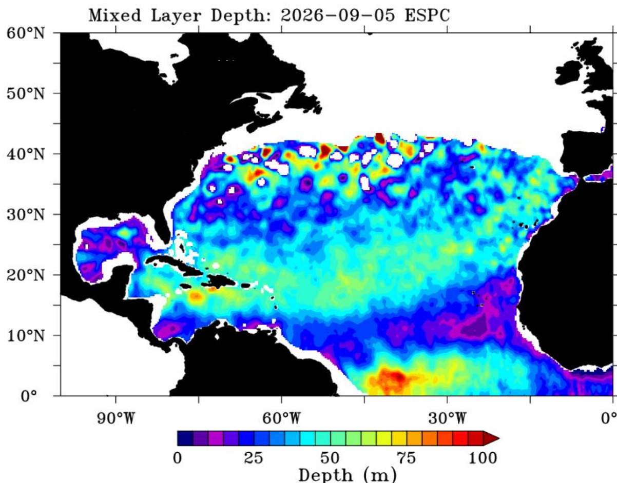
FIGURA 59. Variación en la extensión espacial de la profundidad de la capa mixta del océano. Fuente: https://www.ospo.noaa.gov/Products/ocean/ohc/ (accedido: 5 de septiembre de 2026).
