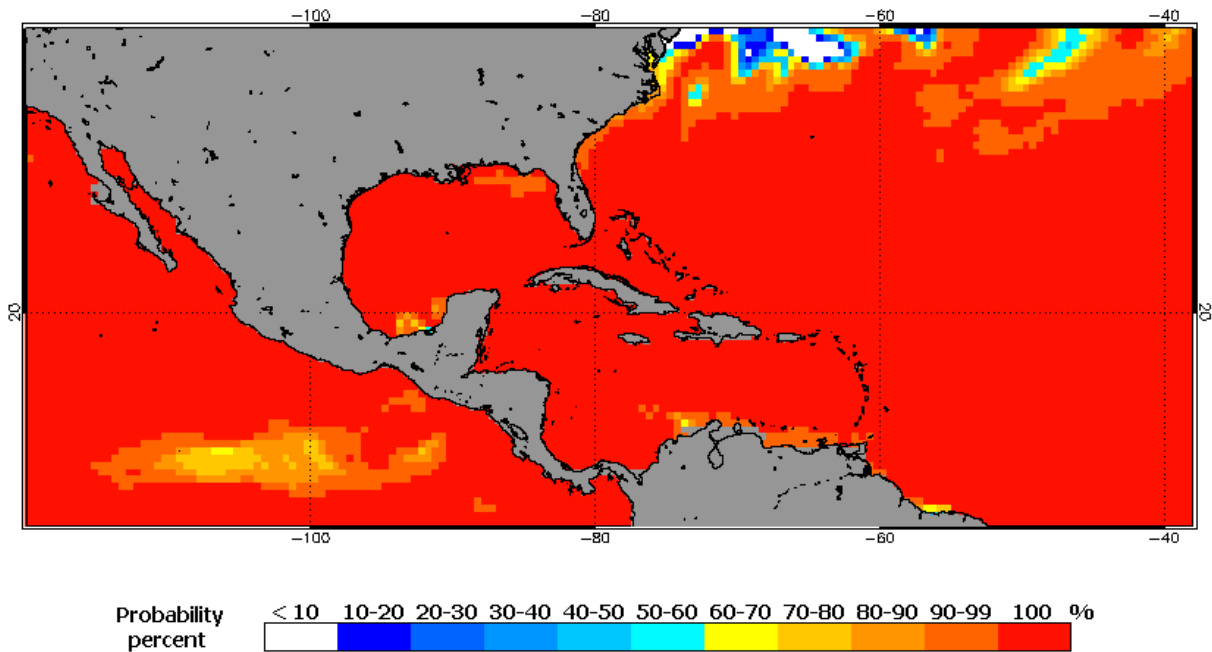
FIGURA 52. Proyección de probabilidad de emisión de al menos una vigilancia o mayor de blanqueamiento inminente de los corales en el Caribe para el periodo de septiembre a diciembre de 2026. Accedido: 5 de septiembre de 2026. Fuente: https://coralreefwatch.noaa.gov/satellite/bleachingoutlook_cfs/current_image/cur_cfsv2_prob-4mon_v5_watch_caribbean.gif
