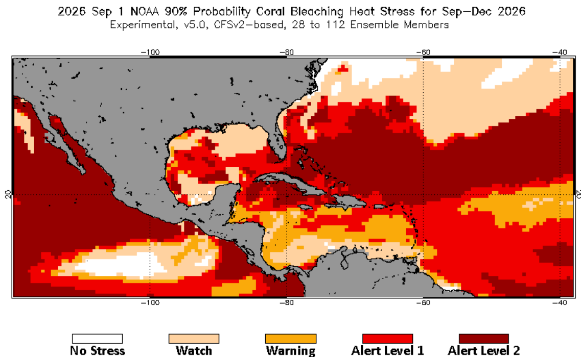
FIGURA 47. Proyección de probabilidad de 90% o mayor de estrés térmico conducente al blanqueamiento de los corales en el Caribe para el período de septiembre a diciembre de 2026. Accedido: 5 de septiembre de 2026. Fuente: https://coralreefwatch.noaa.gov/satellite/bleachingoutlook_cfs/current_image/cur_cfsv2_outlook-4mon_v5_90pct_caribbean.gif
