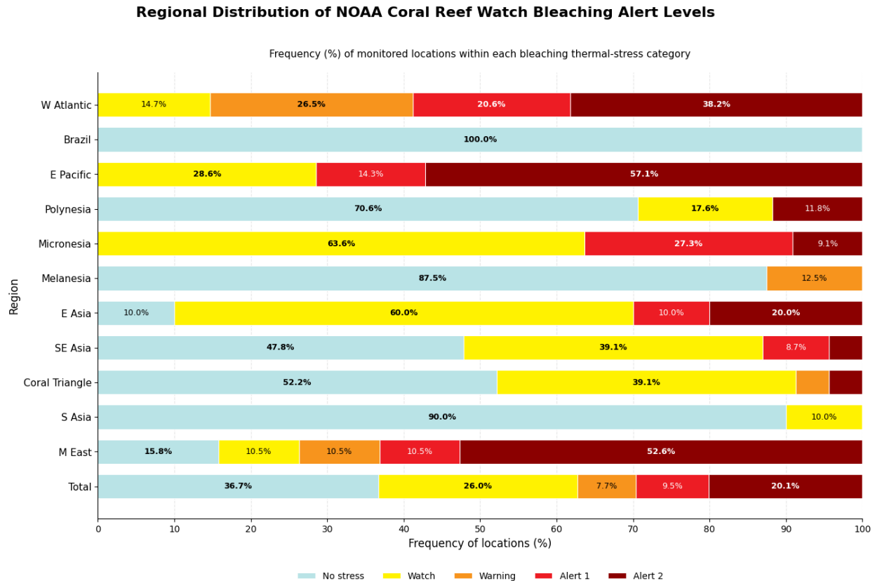
FIGURA 53. Clasificación de riesgos de blanqueamiento de corales a través de 11 regiones del planeta (N=169 estaciones de monitoreo de temperatura del agua. Fuente: https://coralreefwatch.noaa.gov/product/vs/data.php (accedido: 5 de septiembre de 2026).
