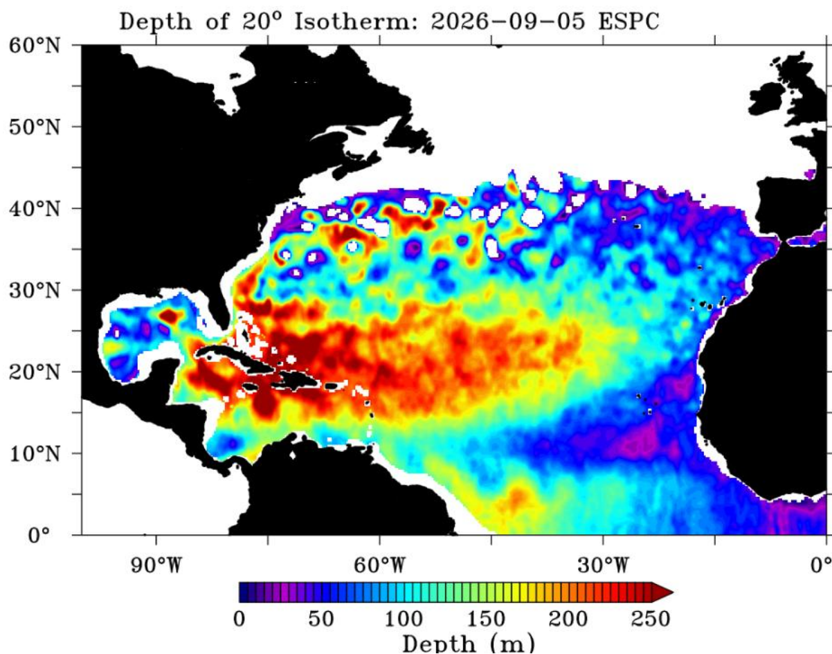
FIGURA 61. Variación en la extensión espacial de la profundidad de la isoterma oceánica de 20°C. Fuente: https://www.ospo.noaa.gov/Products/ocean/ohc/ (accedido: 5 de septiembre de 2026).
