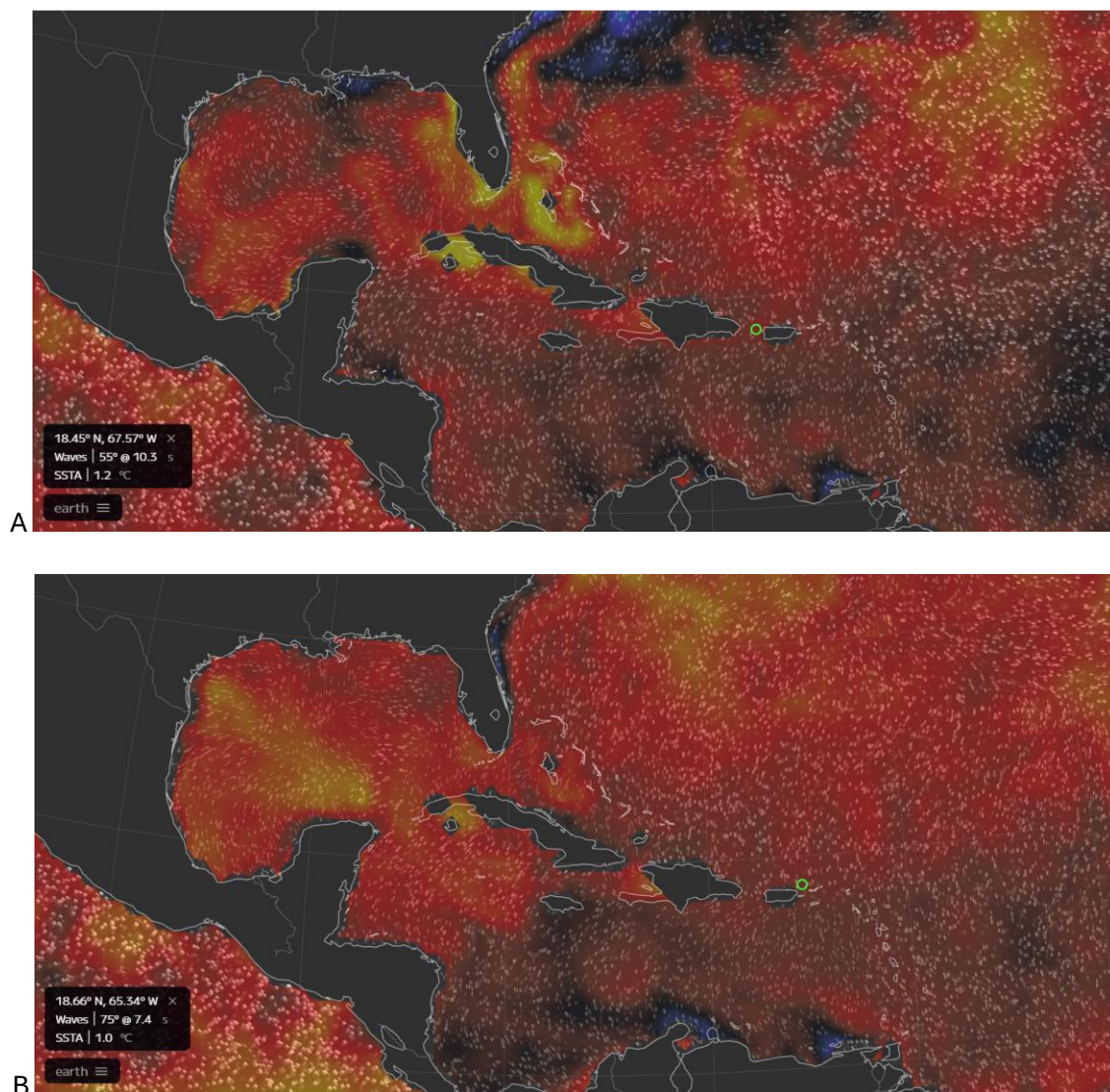
FIGURA 9. Imagen en tiempo real de las anomalías térmicas de la superficie del mar en zona del Caribe. Accedido: A) 13 de mayo de 2026; B) 5 de septiembre de 2026. Fuente: https://earth.nullschool.net/#current/ocean/primary/waves/overlay=sea_surface_temp_anomaly/orthographic=-76.54,19.90,1797/loc=-65.389,18.208
