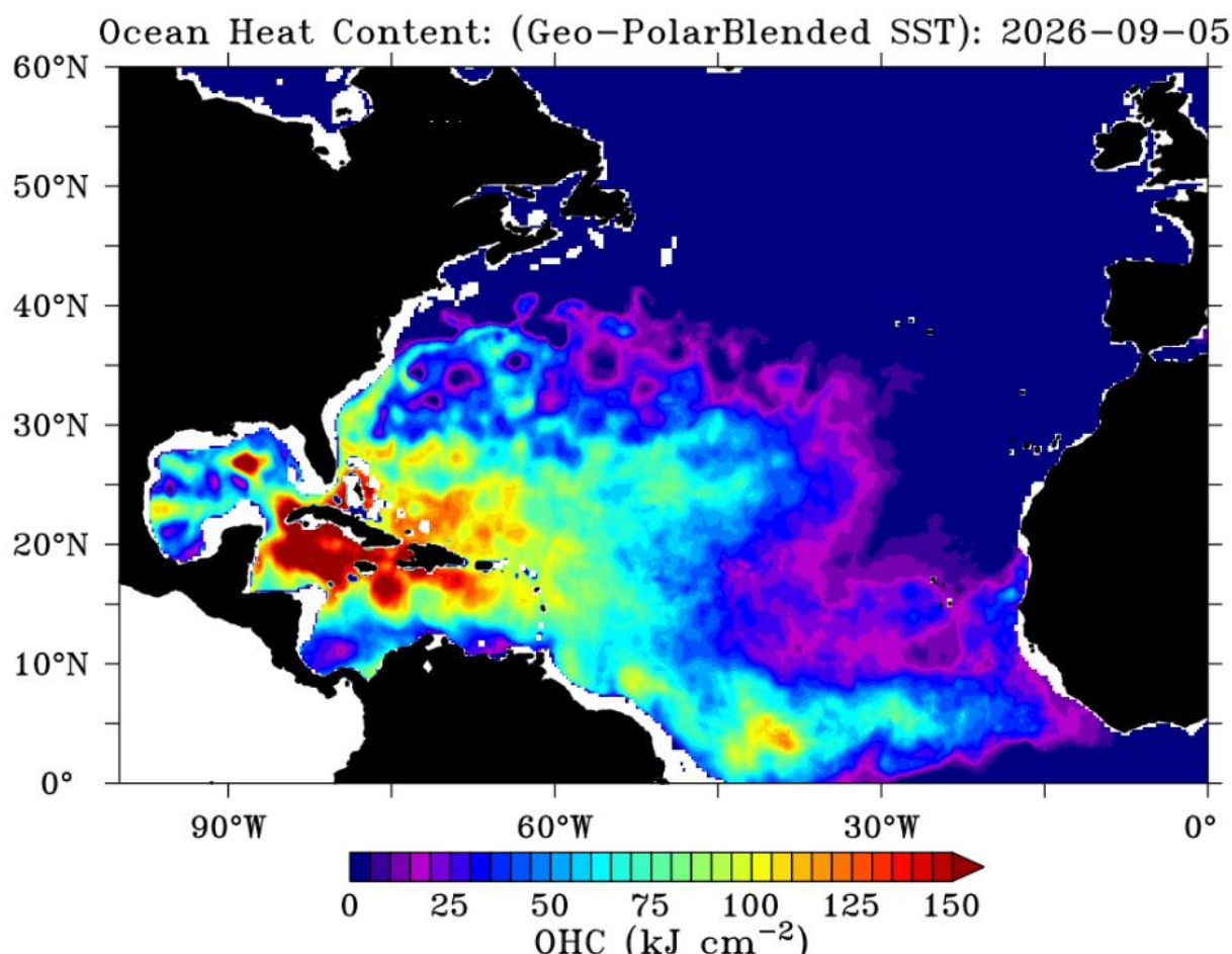
FIGURA 54. Extensión espacial del contenido de calor del océano a comienzos de septiembre de 2026. Fuente: https://www.ospo.noaa.gov/Products/ocean/ohc/ (accedido: 5 de septiembre de 2026).
