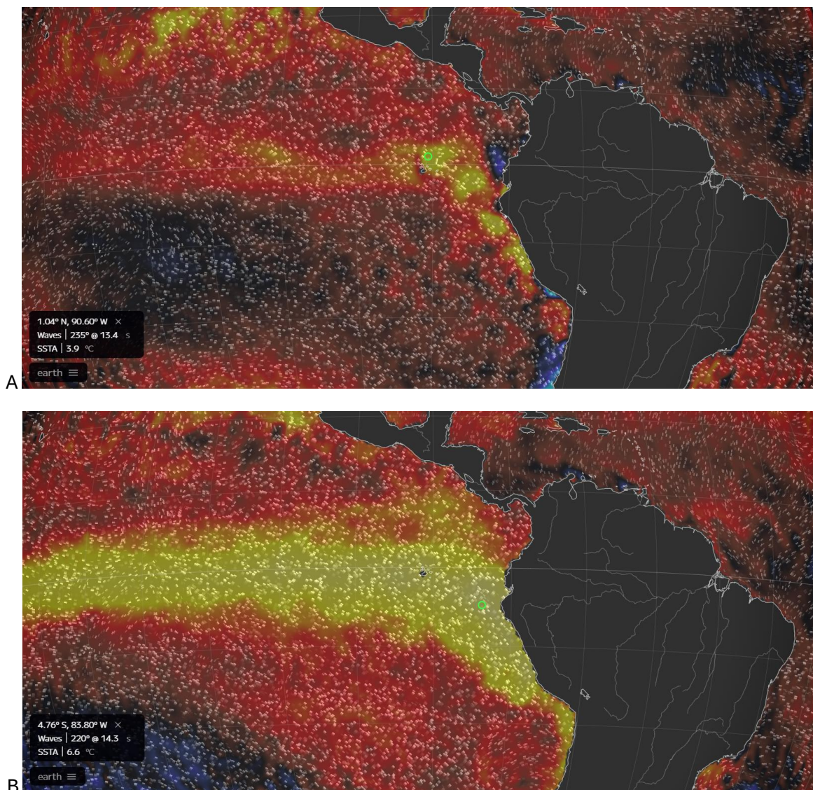
FIGURA 8. Imagen en tiempo real de las anomalías térmicas de la superficie del mar en zona este del Pacífico tropical, en la costa oeste de Sur América. Accedido: A) 13 de mayo de 2026; B) 5 de septiembre de 2026. Fuente: https://earth.nullschool.net/#current/ocean/primary/waves/overlay=sea_surface_temp_anomaly/orthographic=-91.89,-4.38,894/loc=-83.649,-2.865
