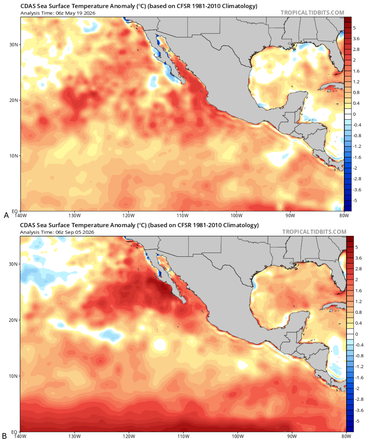
FIGURA 11. Patrones de distribución de las anomalías térmicas en la superficie del mar en el este del Pacífico tropical. Accedido: A) 19 de mayo de 2026; B) 5 de septiembre de 2026. Fuente: https://www.tropicaltidbits.com/analysis/ocean/cdas-sflux_ssta_epac_1.png
