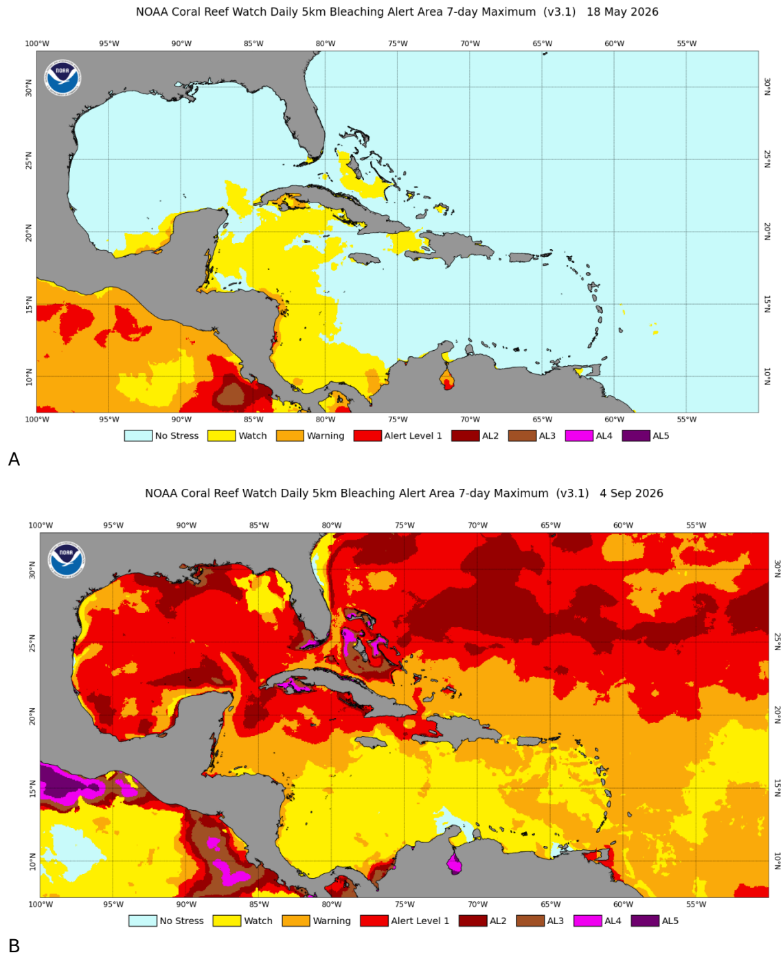
FIGURA 44. Areas bajo alertas de blanqueamiento de corales en el Caribe, basado en el NOAA Coral Reef Watch Program. Accedido: A) 19 de mayo de 2026; B) 5 de septiembre de 2026. Fuente: https://coralreefwatch.noaa.gov/data_current/5km/v3.1_op/daily/png/ct5km_baa5-max-7d_v3.1_caribbean_current.png
